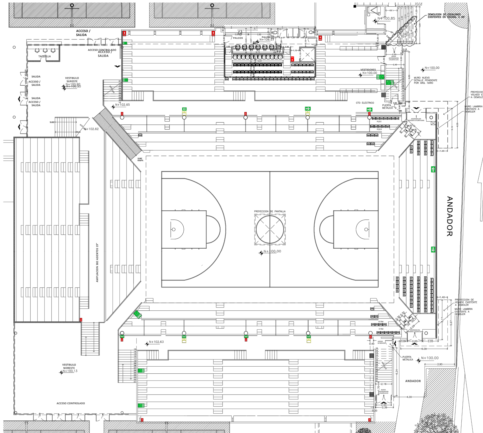
PLANTA ARQUITECTONICA ALTA DE UBICACION DE SIMBOLOGIA PARA PROTECCION CIVIL.
